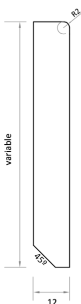
Rodapié recto 9 E=1/2 Cotas mm
