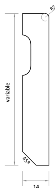
Rodapié recto 12 E=1/1 Cotas mm
