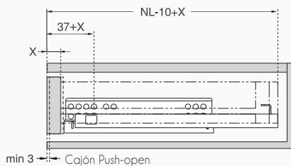
NL = Largo Nominal Lateral LT = Profundidad interna del módulo LT = NL + X
