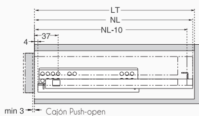
NL = Largo Nominal LT = Profundidad interna del módulo LT = NL + 3
