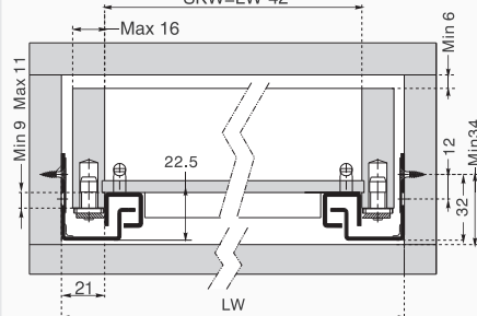
SKW = Ancho interior del cajón LW = Ancho interior del módulo SKW=LW-42
