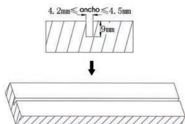
1. Ranurado como se muestra.
