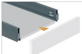
2_ Colocar el frontal
